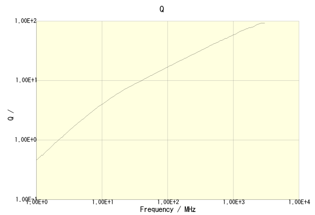
MLG1608B4N7ST000
