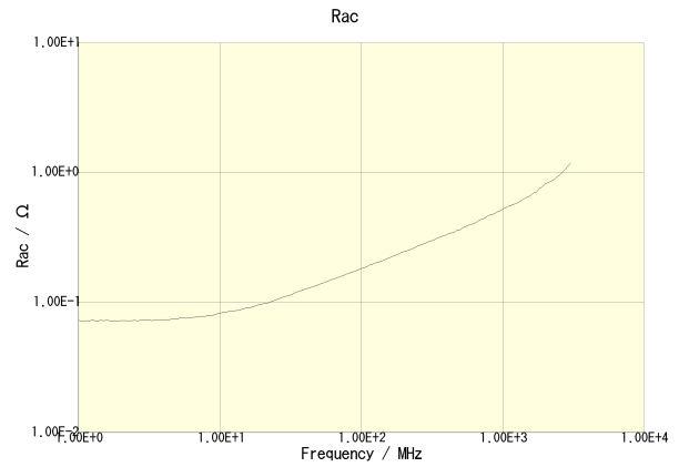
MLG1608B4N7ST000
