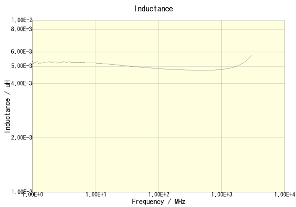
MLG1608B4N7ST000
