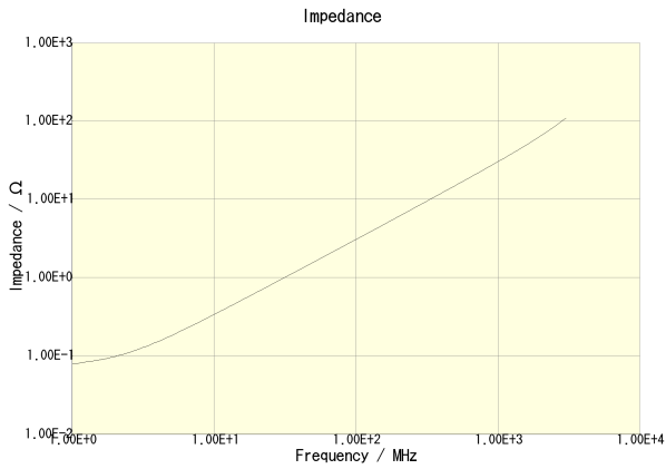
MLG1608B4N7ST000
